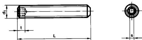
DIN 913 / ISO 4026 (flat point)
